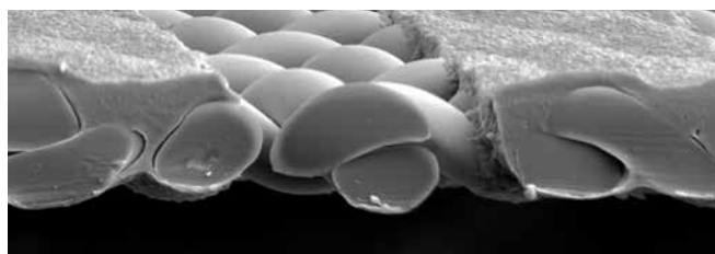
SEFAR® PET 1500 180/460-27Y, emulsione diretta con 4 µm EOM
