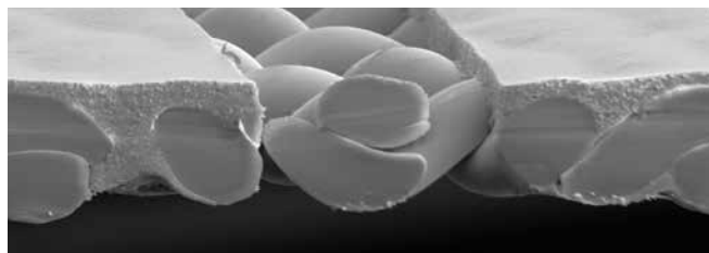
Canale di stampa rettangolare, bordi nitidi con SEFAR® PCF FC 180/460-27Y, 3 µm EOM
