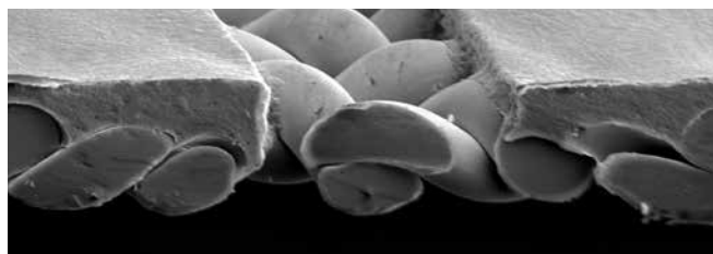
SEFAR® PET 1500 180/460-27Y, film capillare 15 con 7 µm EOM
