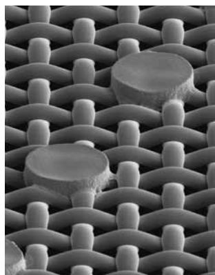
Adesione della matrice di SEFAR® PET 1500 120/305-34Y
