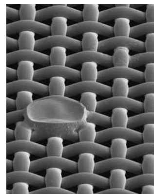
Adesione della matrice di un normale tessuto di poliestere 120/305-34Y
