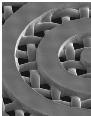
Protezione alla diffusione della luce UV di SEFAR® PET 1500 120/305-34Y
